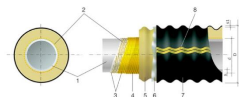
1. Тонкостенная труба РЕХ-а. 2. Армировка из арамидного волокна Кевлар®. 3. Последовательность слоев из сополимеров этилена. 4. Кислородно-защитный слой. 5. Теплоизоляция из полужесткого ППУ. 6. Барьерный слой. 7. Защитная оболочка из полиэтилена. 8. Идентификационные полосы желтого цвета.
