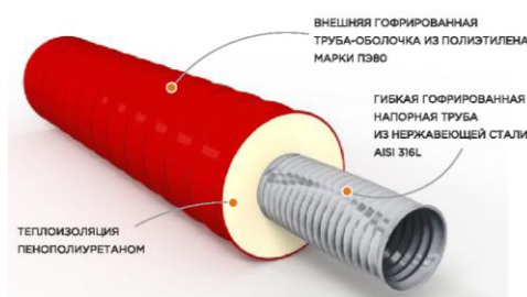
Гибкие системы трубопроводов в ППУ изоляции
